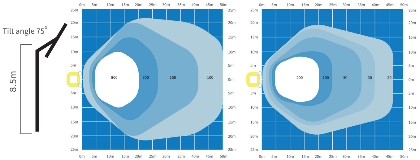
IWE-PL6K-480 - 480 000 Lumens 4 Lights - Verticle
